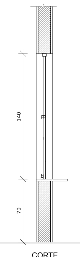
J18 QUANT. 01 DIMENSÕES: 140 x 140 cm PEITORIL 70 cm SISTEMA: Fina e Guilhotina AMBIENTE: - Cozinha
