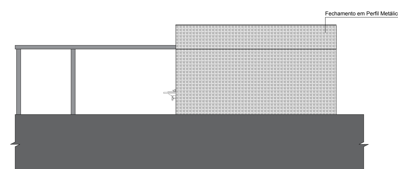
Elevação 16 Esc.: 1/100
