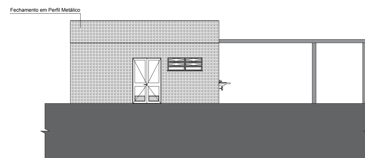
Elevação 15 Esc.: 1/100
