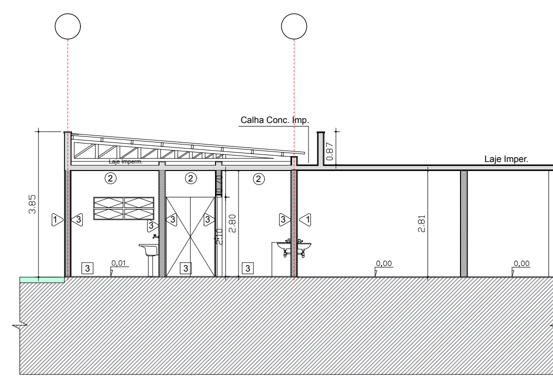
Corte GG Esc.: 1/100
