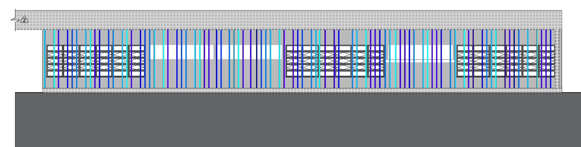
Elevação Fundos (do acesso à área administrativa) Opção com brises Esc.: 1/100
