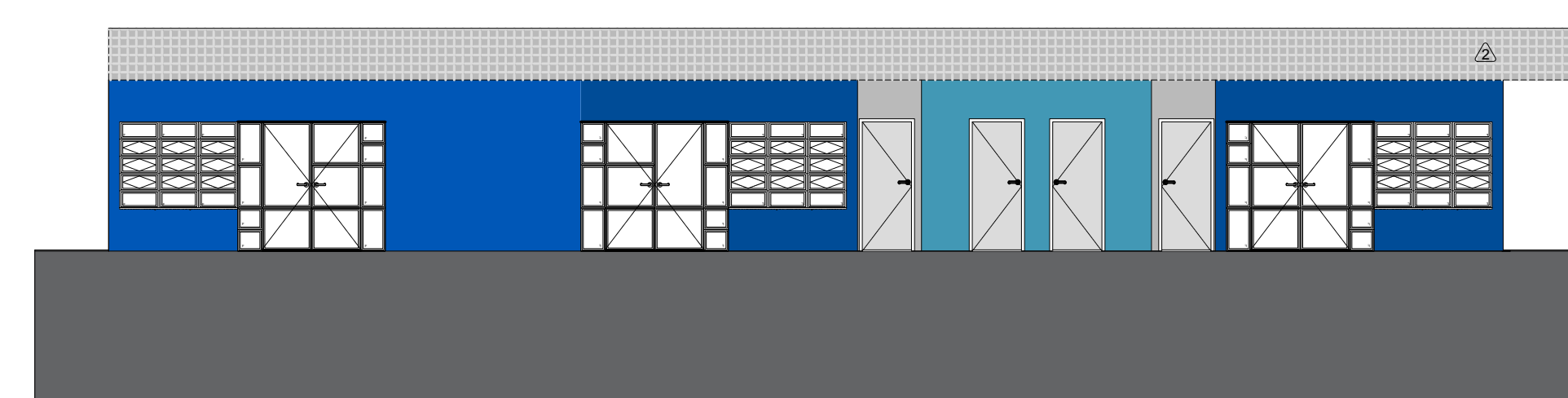
Elevação Frontal (do acesso à área administrativa) Esc.: 1/100
