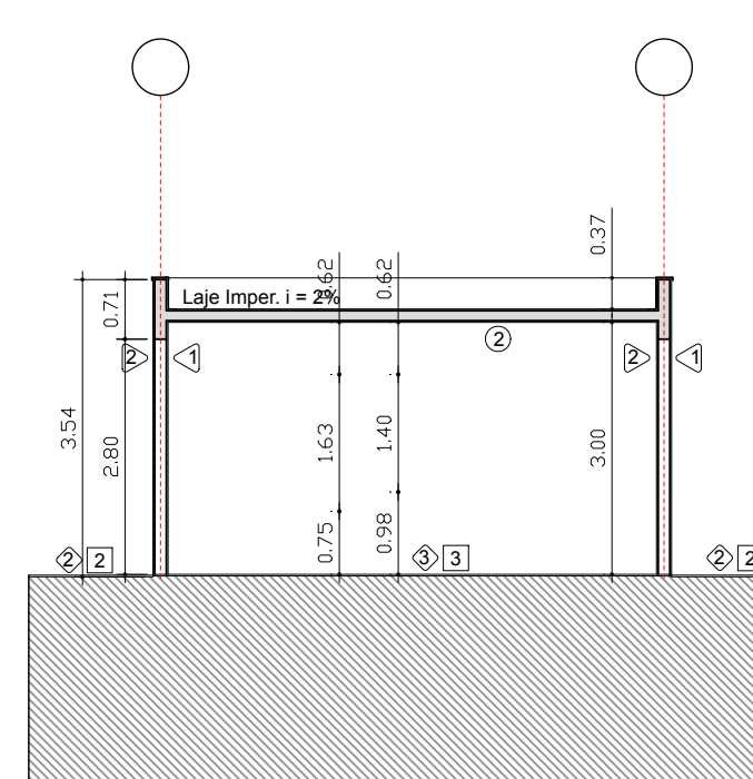
Corte Transversal Secretaria Esc.: 1/100
