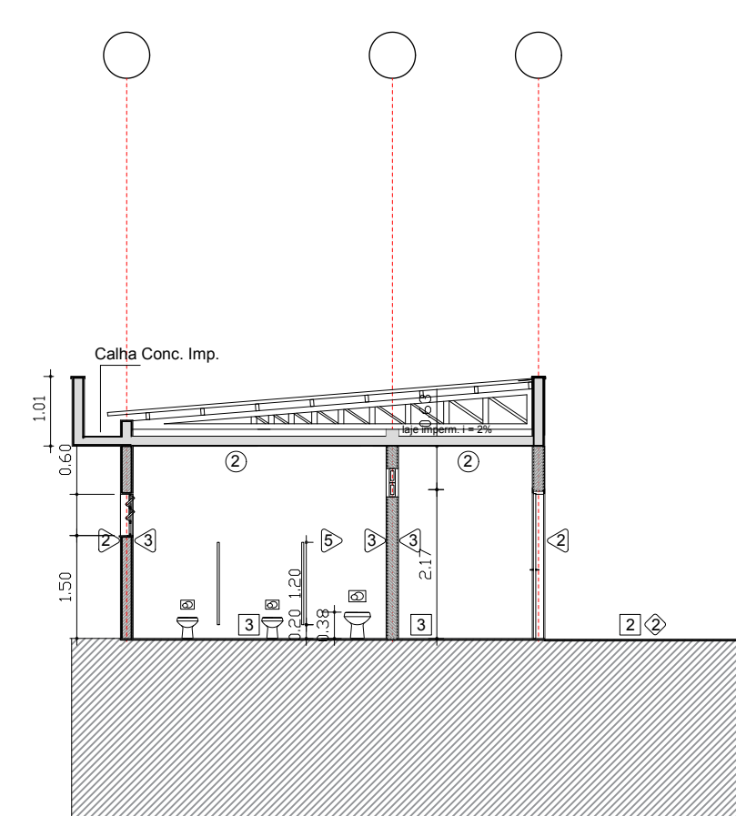
Corte Transversal Esc.: 1/100
