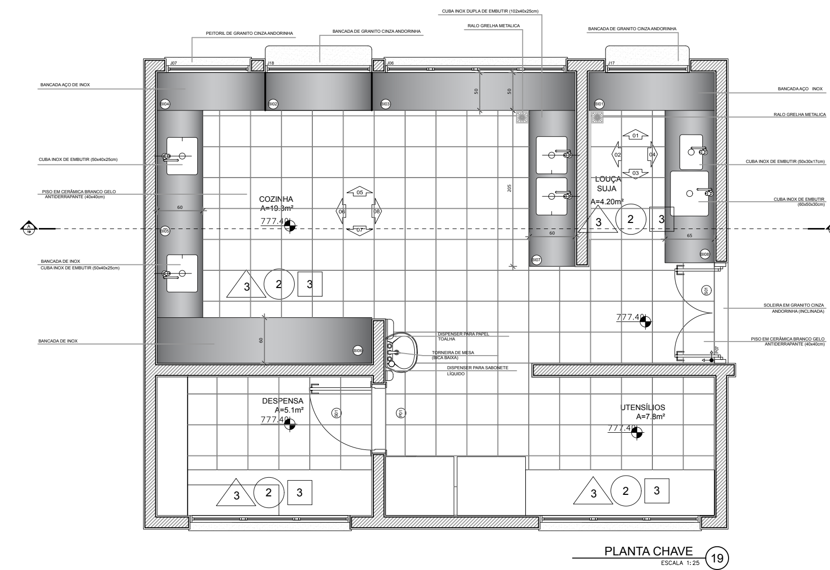
PLANTA CHAVE
