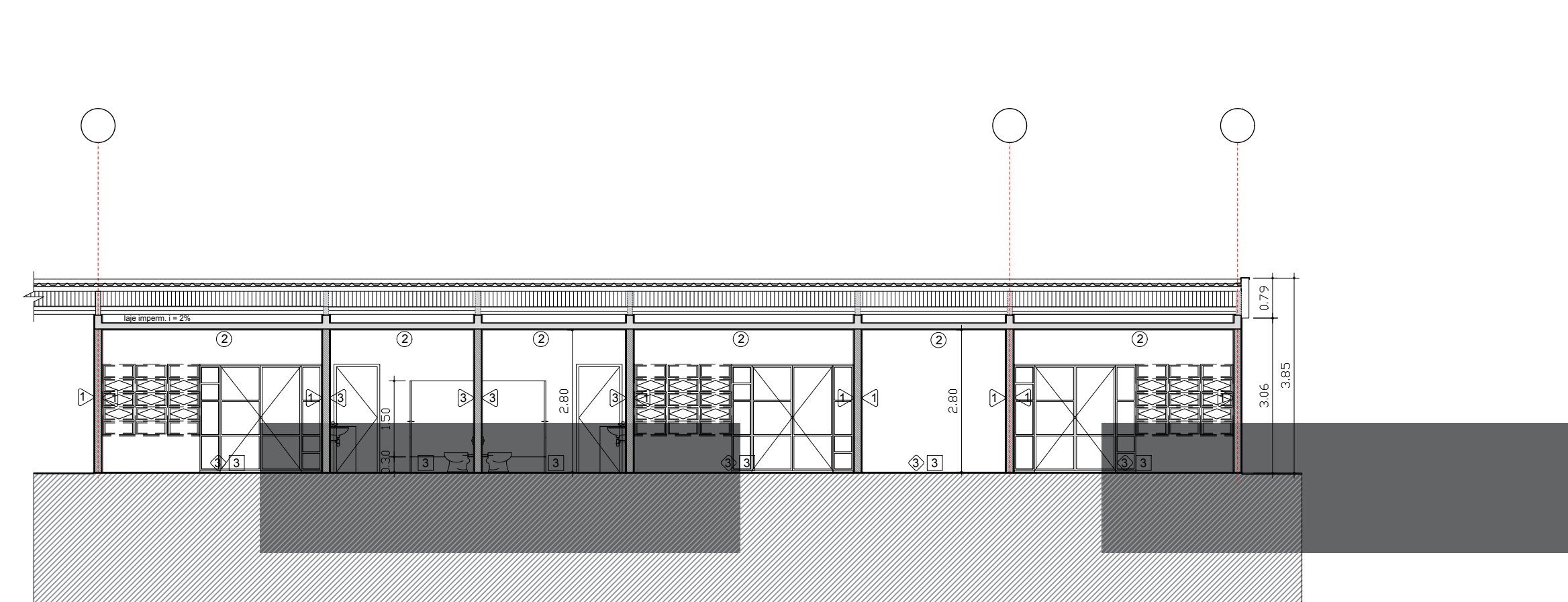
Corte Longitudinal Esc.: 1/100
