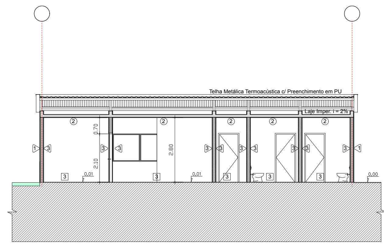
Corte HH Esc.: 1/100
