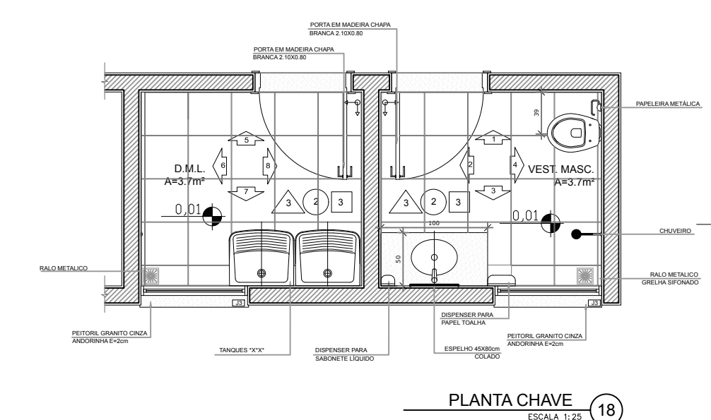
PLANTA CHAVE
