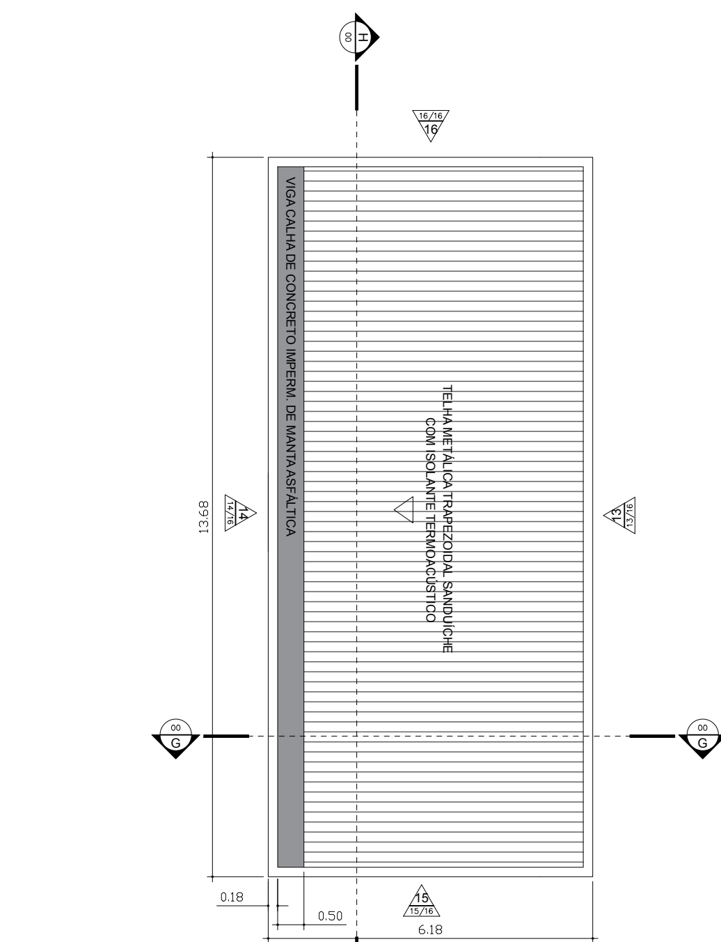
Planta Cobertura Esc.: 1/100
