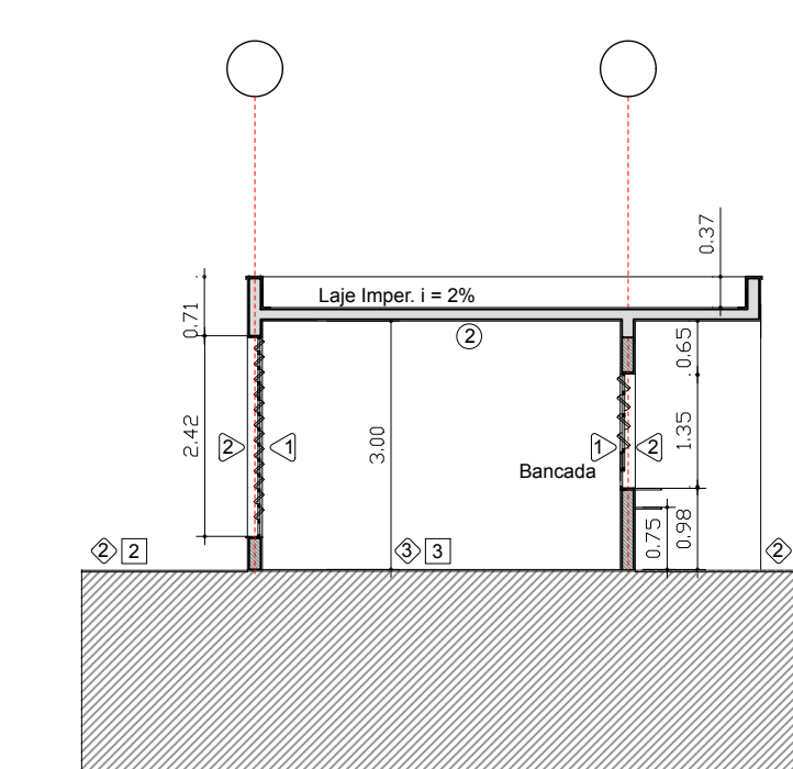
Corte Longitudinal Secretaria Esc.: 1/100
